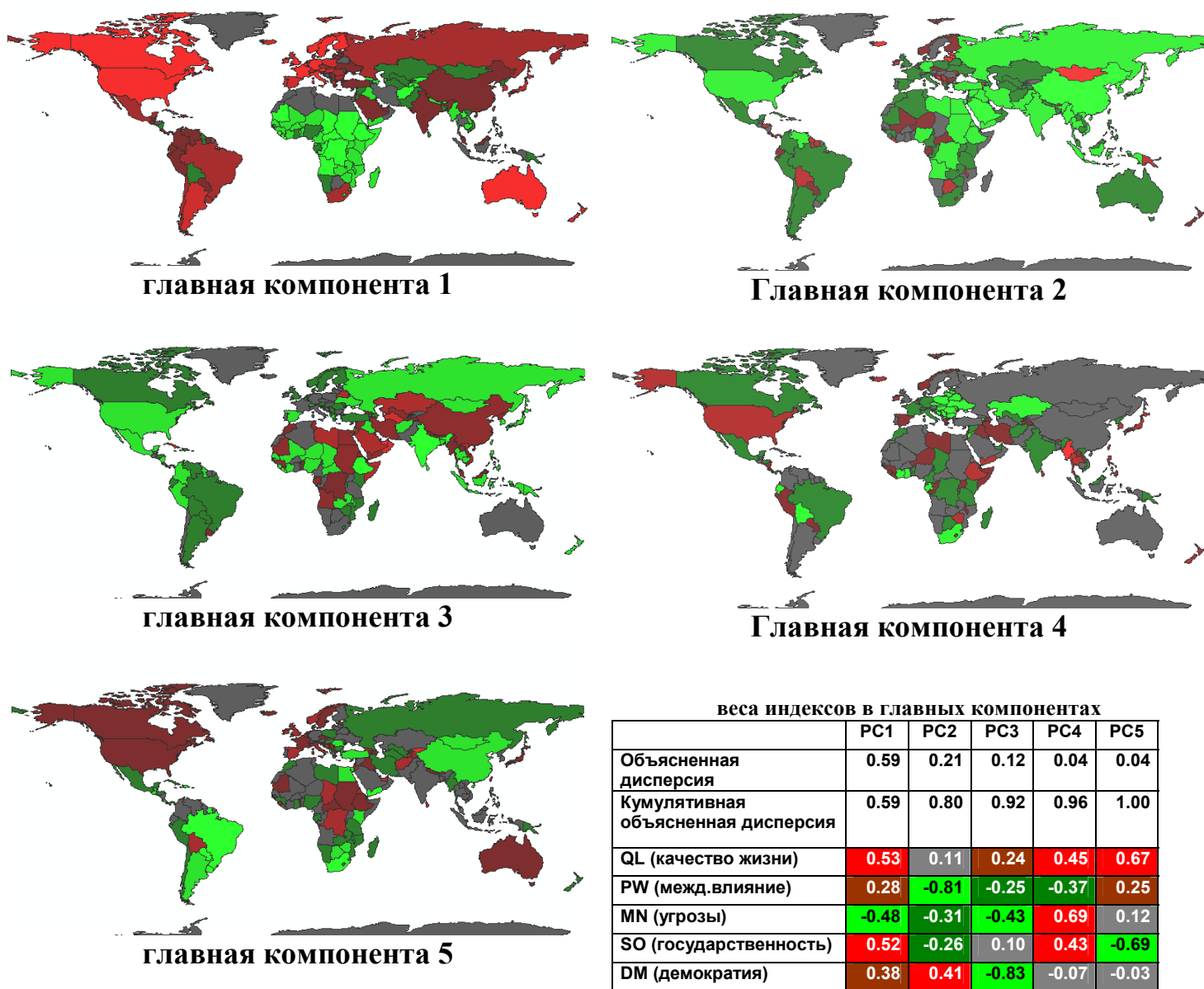
Рис. 2. Анализ главных компонент данных рейтингов “Политического Атласа Современности” и визуализация проекций (нагрузок) стран на главные компоненты. Красный цвет отображает положительные проекции, зеленый – отрицательные, серый – близкие к нулю, интенсивность цвета пропорциональна абсолютному значению проекции.
